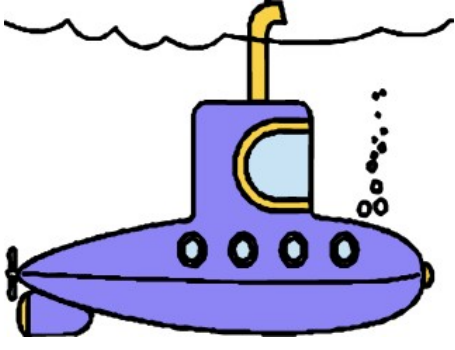
غواصة
