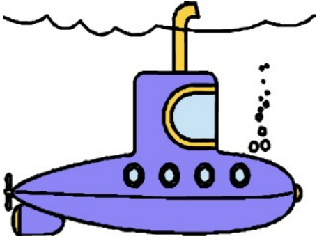
غواصة
